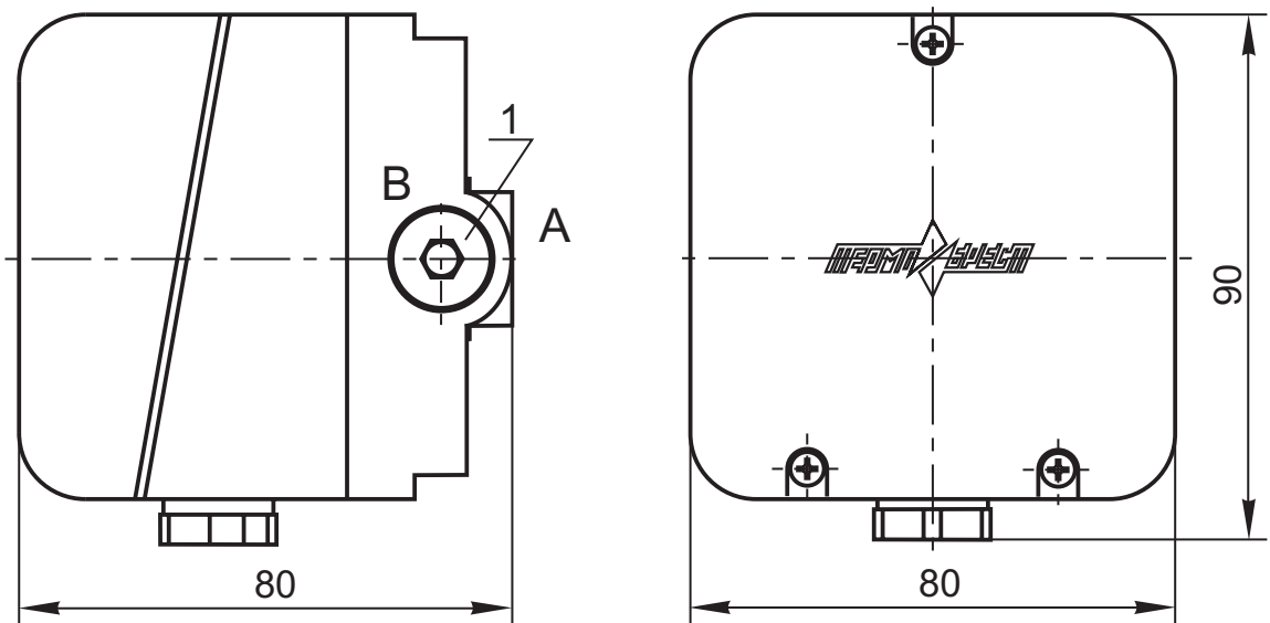
Рис. 23-2. Габаритные размеры датчиков-реле избыточного давления (напора) серии ДРД-Н
