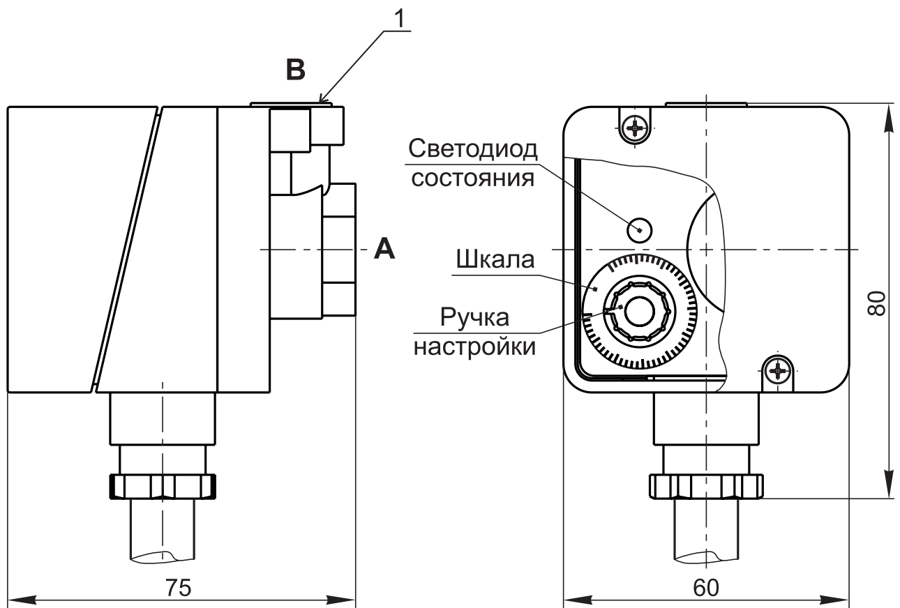
Рис. 23-5. Габаритные размеры датчиков-реле давления серии ДРД электронного типа
