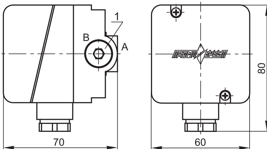
Рис. 23-1. Габаритные размеры датчиков-реле давления серии ДРД
