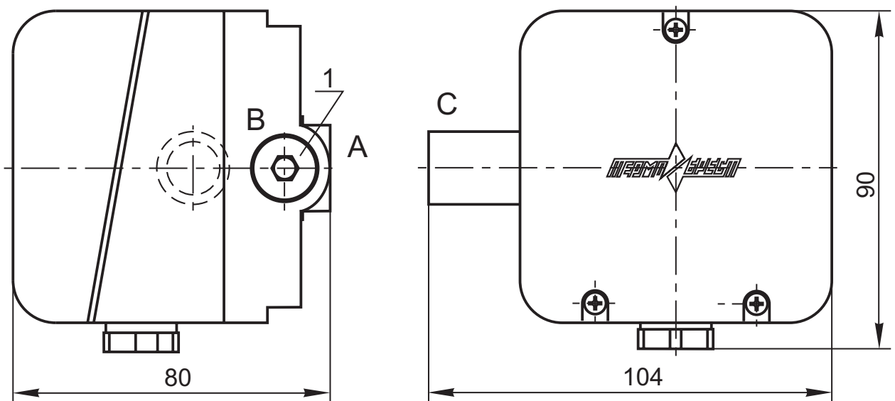
Рис. 23-3. Габаритные размеры датчиков-реле вакуумметрического давления (тяги) серии ДРД-Т
