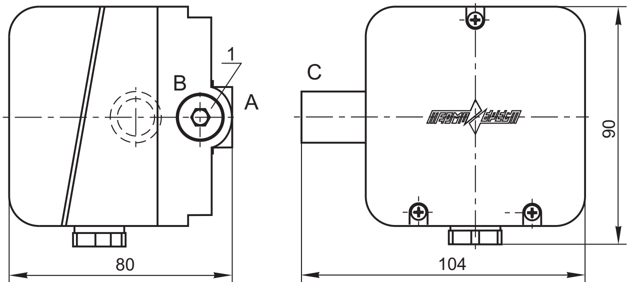
Рис. 23-3. Габаритные размеры датчиков-реле вакуумметрического давления (тяги) типа ДРД-Т
