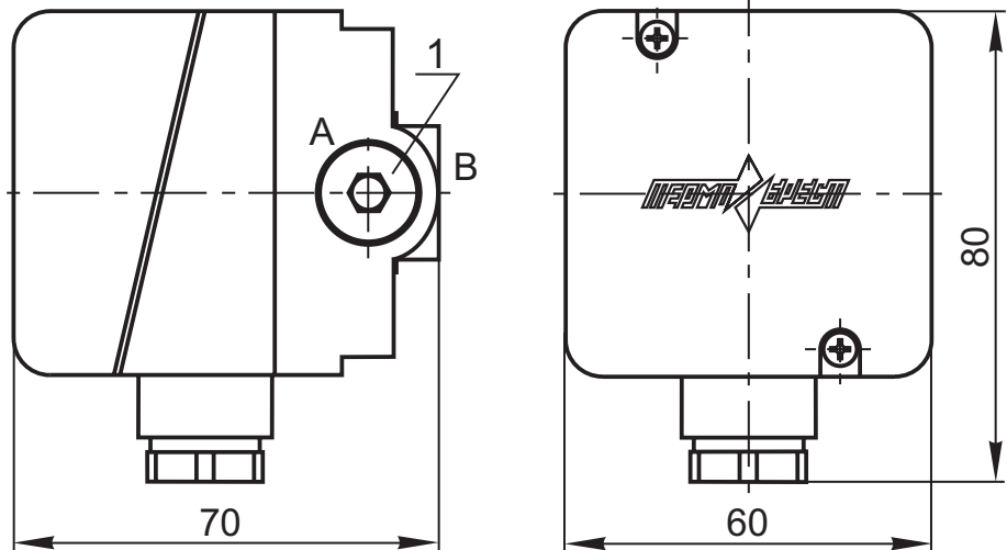
Рис. 23-1. Габаритные размеры датчиков-реле давления типа ДРД
