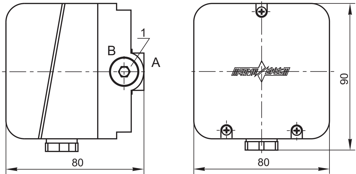
Рис. 23-2. Габаритные размеры датчиков-реле избыточного давления (напора) типа ДРД-Н
